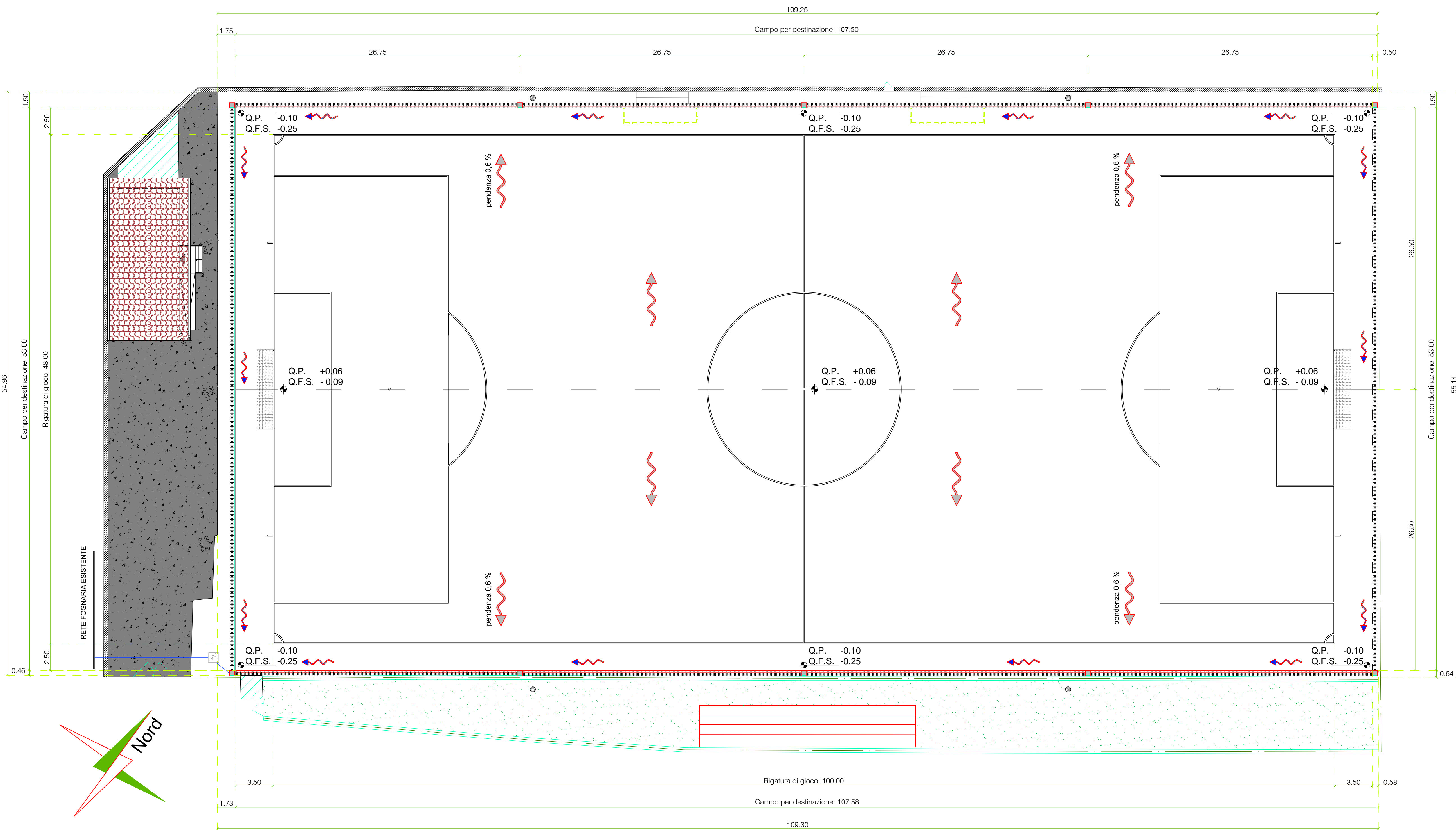
PLANIMETRIA con schema drenaggi e pendenze Scala 1:200
